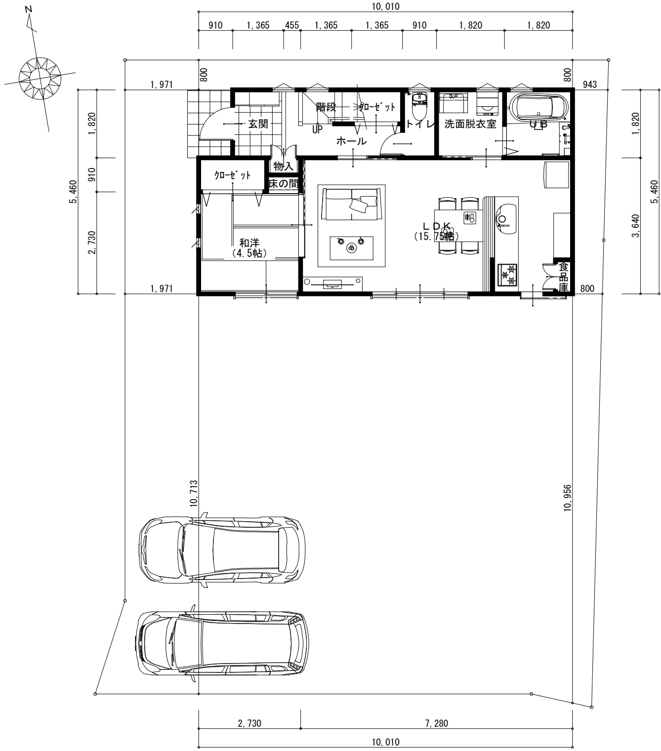
1階 平面図 S:1/100
